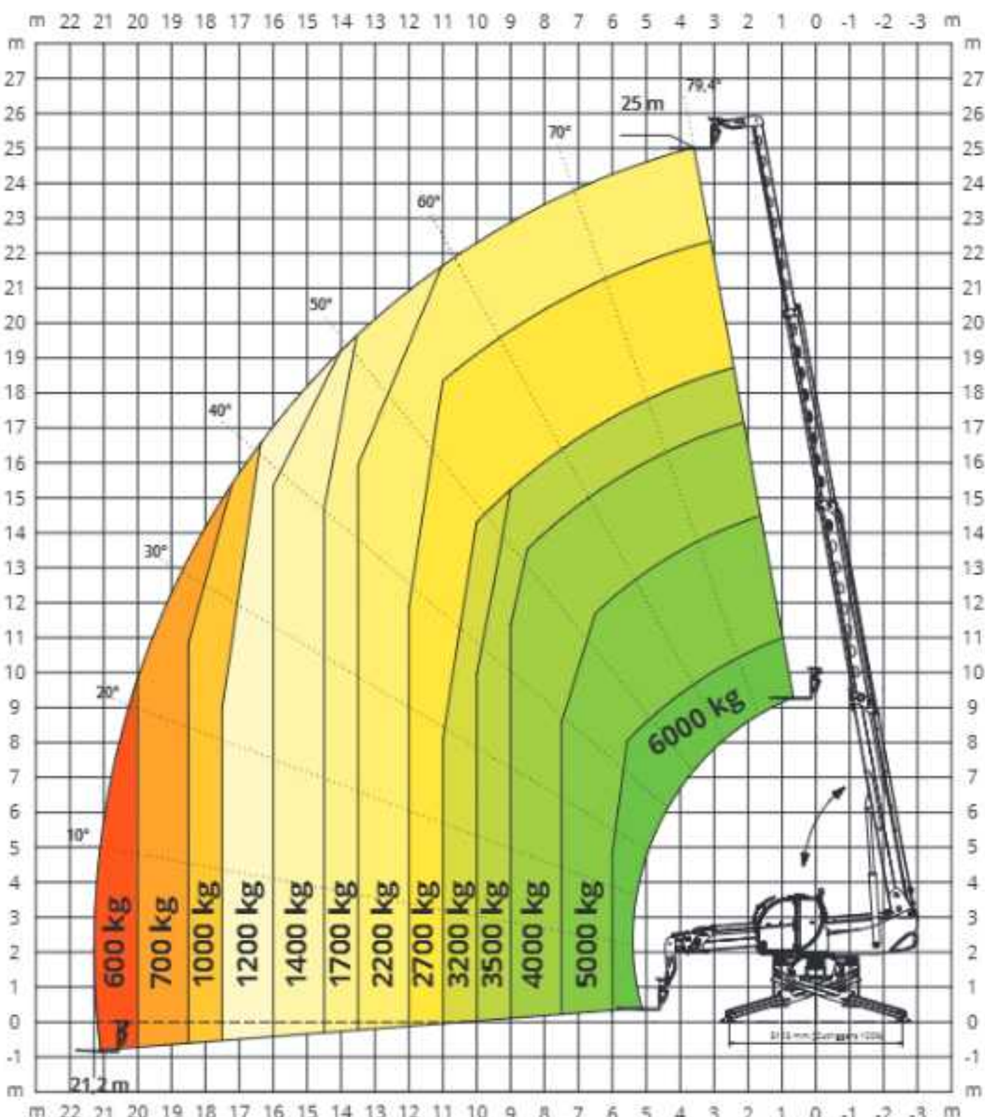
CABRESTANTE 3500 kg
