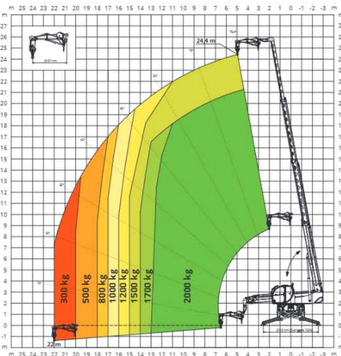
PLUMÍN CON CABRESTANTE 2000 kg
