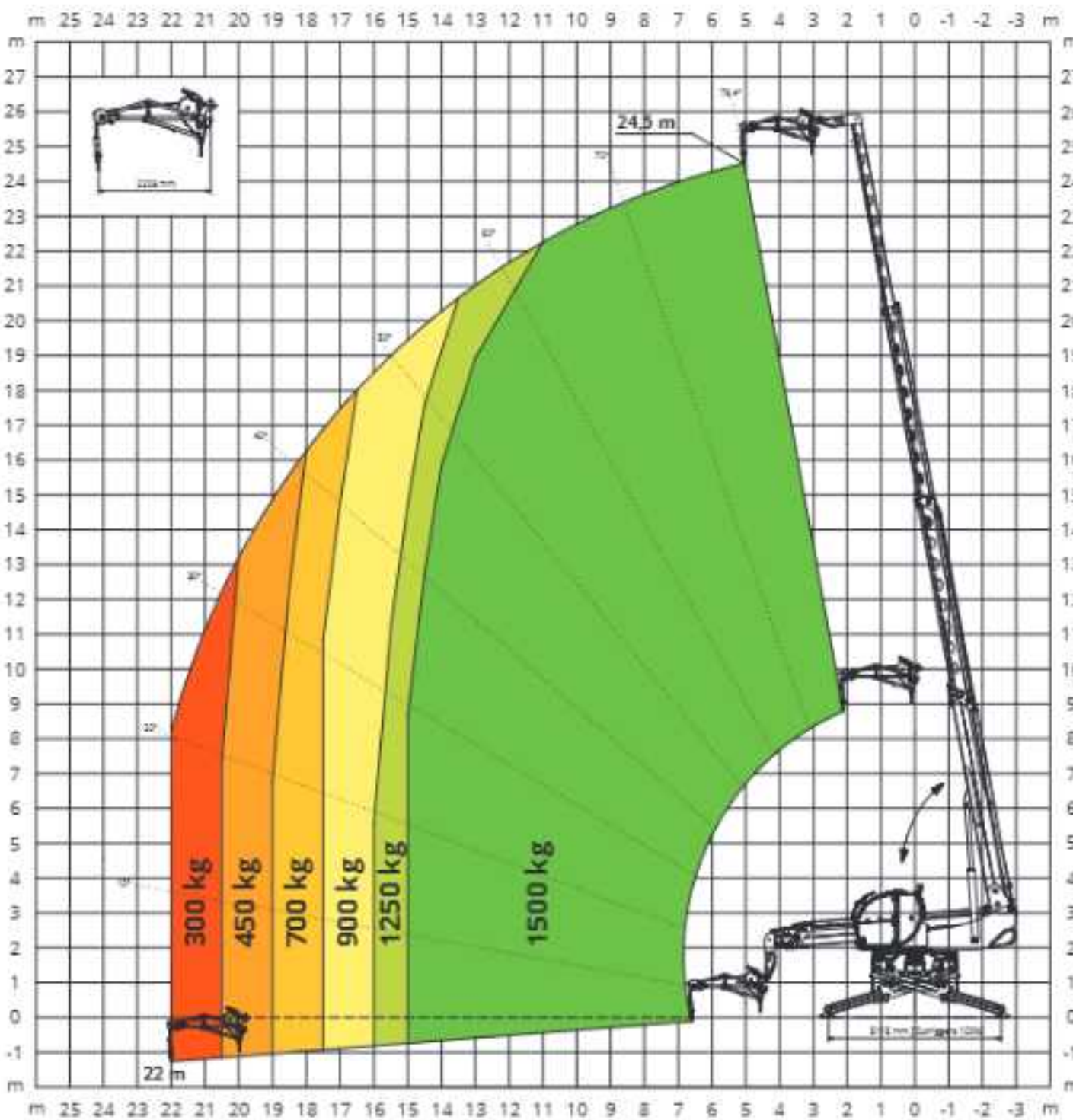
PLUMÍN CON CABRESTANTE 1500 kg
